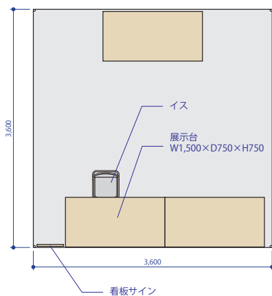
平面図
