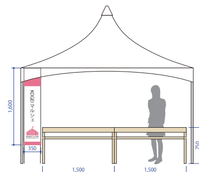
側面図
