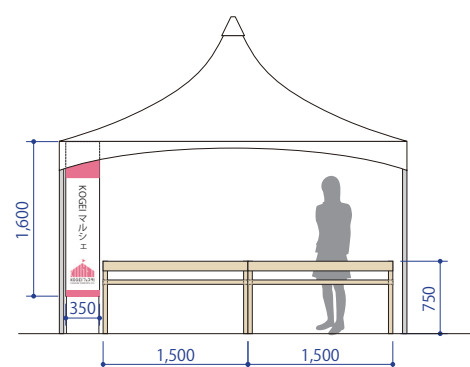
正面図
