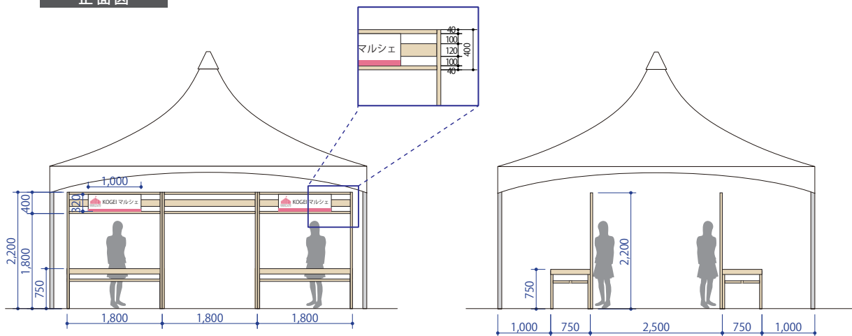
正面図
